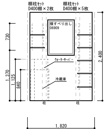
パントリー 南面
