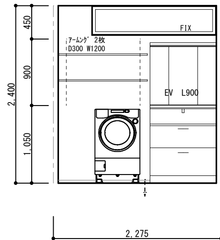
脱衣ラントリー 北面
