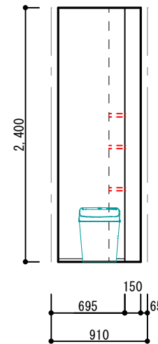
WC① 東面
