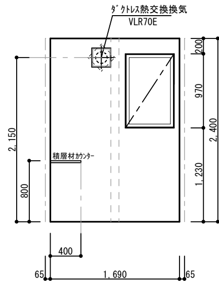
書斎 東面
