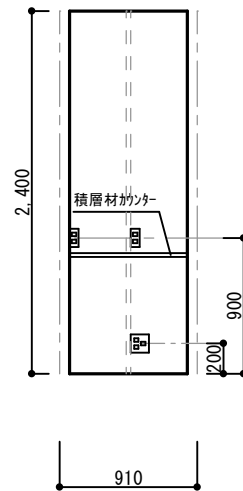
書斎 北面
