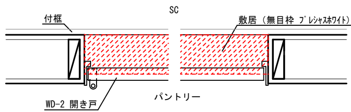
WD-2 建具 納まり図 (1/10)
